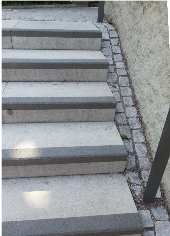
Abb. 3: Detailansicht der Stufen-Vorderkanten-Markierung auf Tritt- und Setzstufen zum Erkennen der Stufen sowohl beim Hoch- als auch beim Runtergehen
